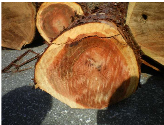
【写真1】伐倒時の衝撃による割れ
